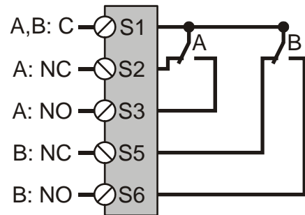
Fig. 14. End switches (Nxx-SW2)
